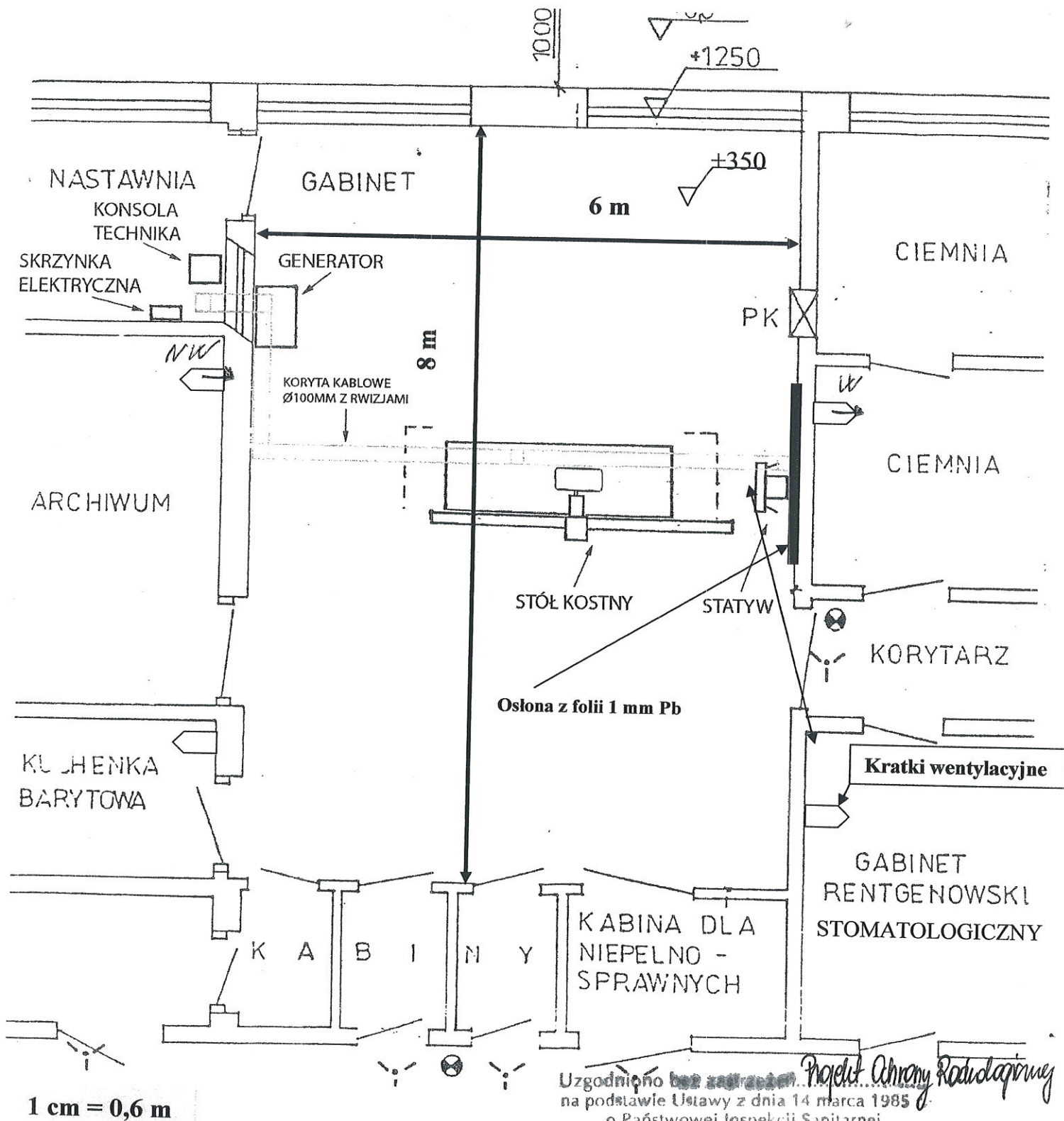
Rysunek 1. Plan gabinetu rtg z projektowanym nowym położeniem aparatu rentgenowskiego.
